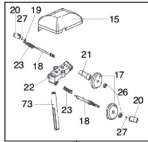
Conjunto afilador Sharpener set Ensemble aigiseur
