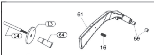
Conjunto brazo pisador Carriage handle set Ensemble poignée du charriot
